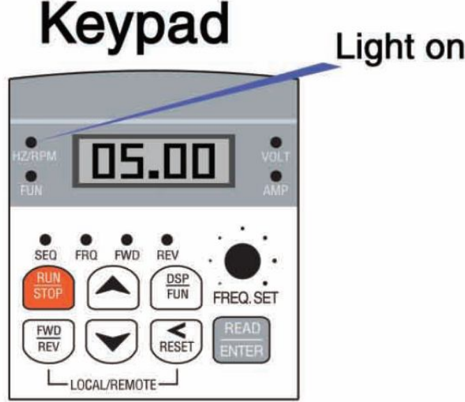
Şekil 4 – İlk açılışta display görünümü
