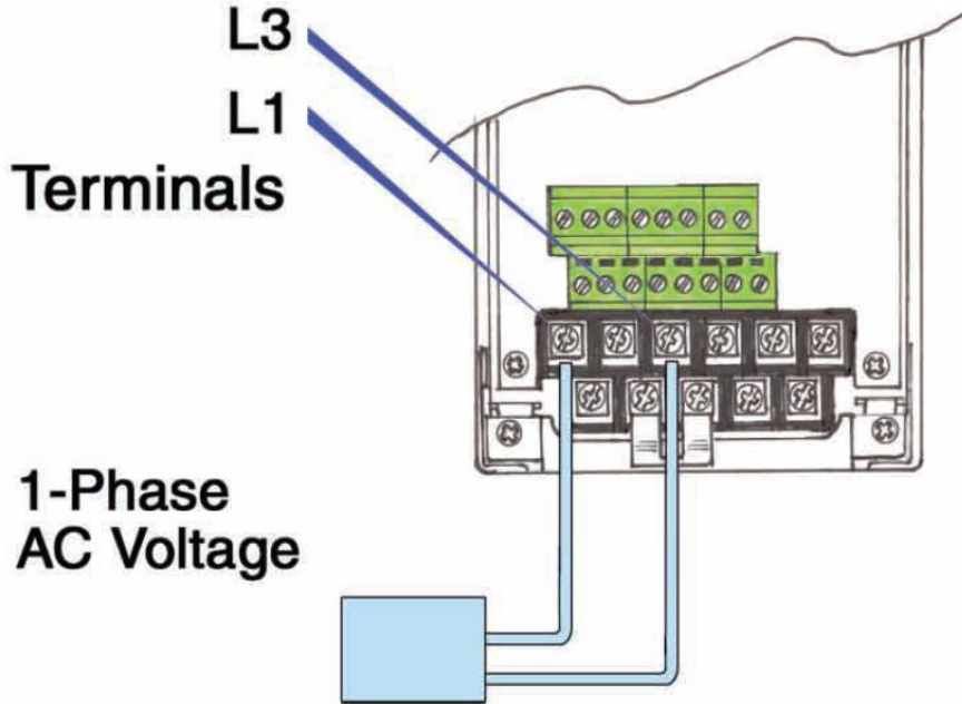
Şekil 1 – Monofaze (220v) Besleme Girişleri gösterimi
