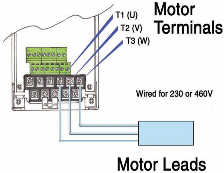
Şekil 3 – Motor Girişleri bağlantısının gösterimi
