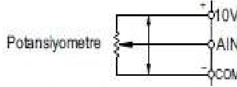
Şekil 5 – Harici Potansiyometre bağlanması
